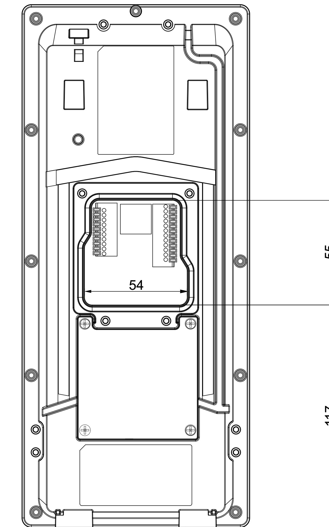
4 后视图
